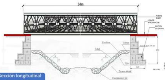
Sección longitudinal Puente Bailey
