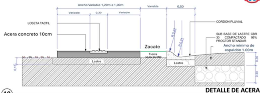
Detalle acera con losa táctil ley 7600 y cordón pluvial
